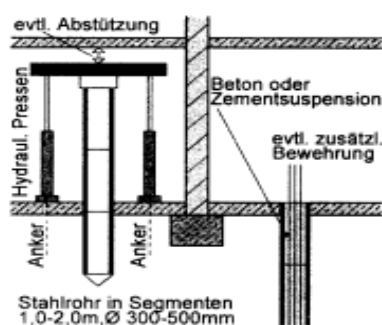
Bild 10, oben: Preßpfahl mit Stahlrohrschüssen, System Franki
