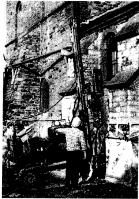
Bild 4: Herstellung der HDI-Säulen unter der Außenwand nach Bild 3 (Werksfoto Bauer, Schrobenhausen)
