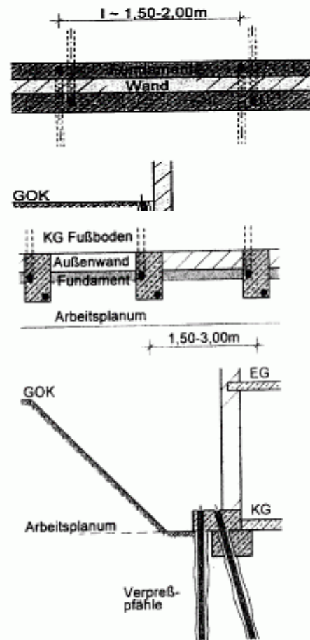
Bild 7: Nachgründung mit kurzem Fundamentbalken, Anordnung außen
