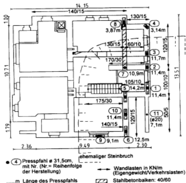
Bild 13: Grundriss mit Anordnung der Segmentpfähle, System Erka
