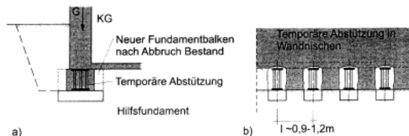
Bild 2: Nachträgliche Herstellung eines Stahlbetonbalkens mit durchgehender Bewehrung a) Systemschnitt, Einbau von punktuellen Abstützungen in Wandnischen b) Ansicht der Hilfsabstützung einer Außenwand
