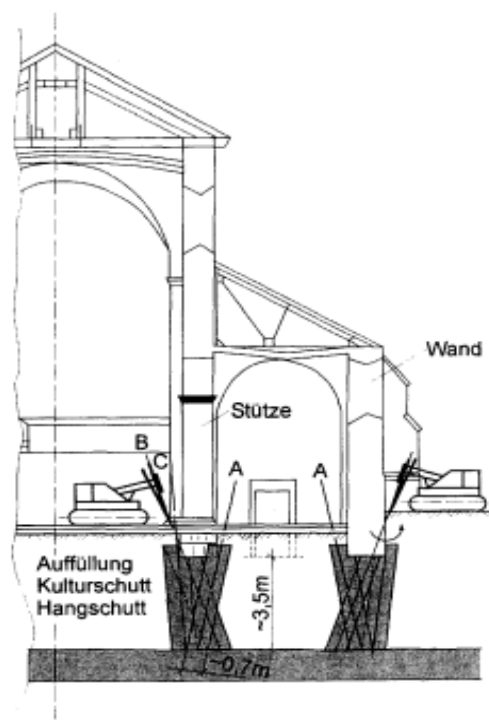
Bild 3: Nachgründung einer Kirche mit dem Düsenstrahlverfahren
