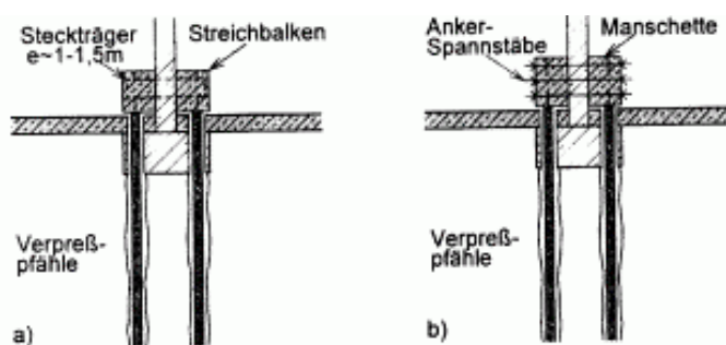
Bild 8: Nachgründung mit beidseitig vertikalen Pfählen a) Streichbalken mit Steckträger b) Manschette und Spannstäbe
