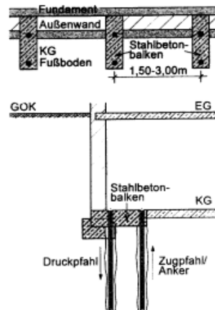
Bild 9: Nachgründung mit Abfangbalken Druck- und Zugpfähle
