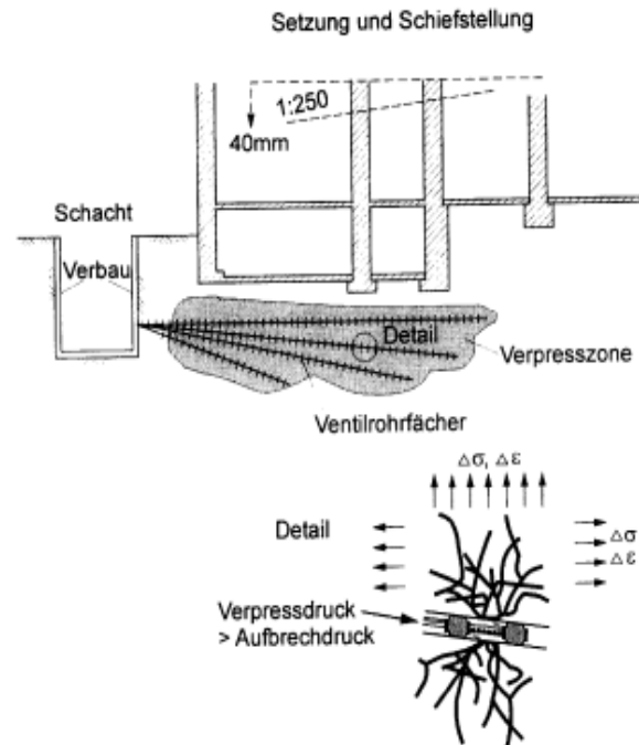
Bild 5: Hebungsinjektion, Erhöhung der Boden-spannung und Hebung durch mehrmaliges Verpressen von Zementsuspension oberhalb des Aufbrechdruckes
